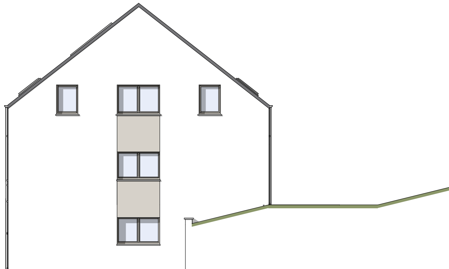
FACADE GAUCHE
