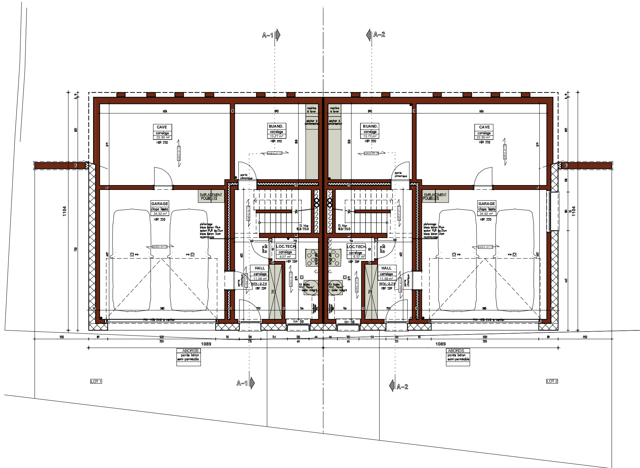
PLAN SOUS-SOL
